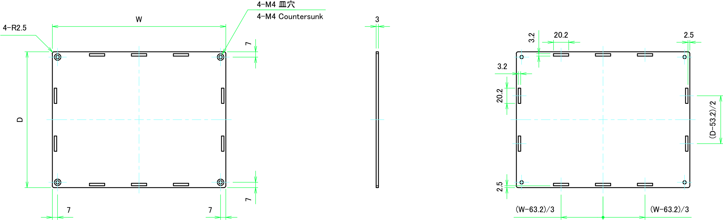
上カバー裏面 / Top cover Backside
