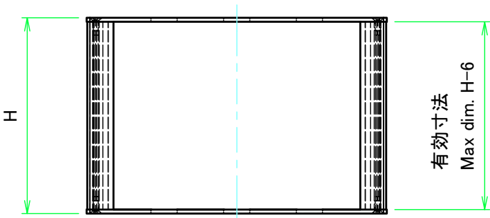
Wパネル1 / W Panel 1
