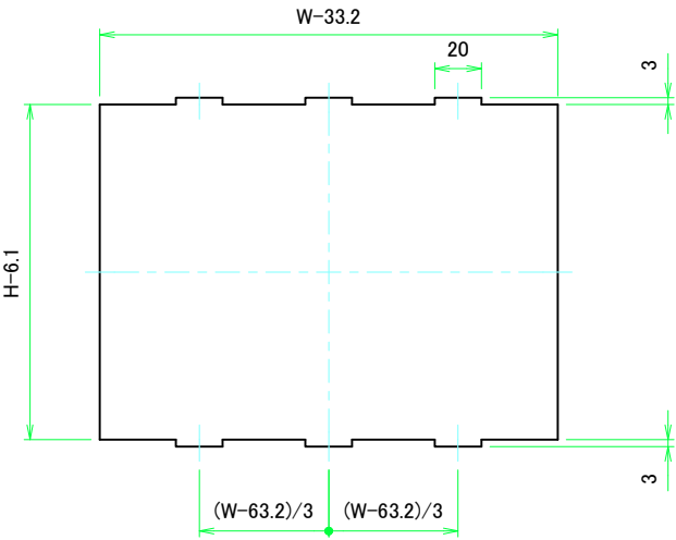
Wパネル1表面 / W Panel 1 Frontside
